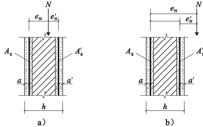
图 5.2.3 加固后的偏心受压构件
