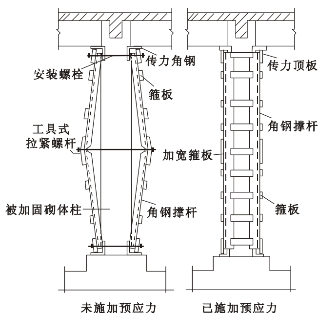
图 8.1.1 预应力撑杆加固方式
