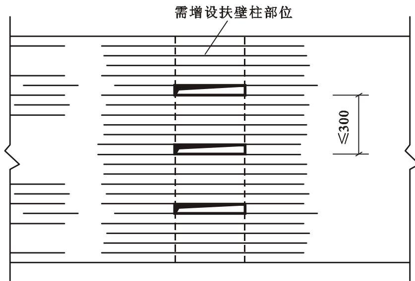
图 10.2.4 水平槽口
